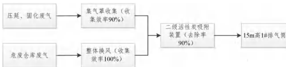
图 4-1 废气污染防治措施一览表
