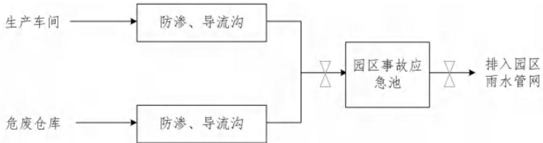
图 4-1 三级防控体系示意图
