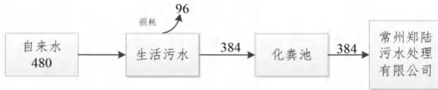
图 2-1 本项目水平衡图 单位：m 3 /a
